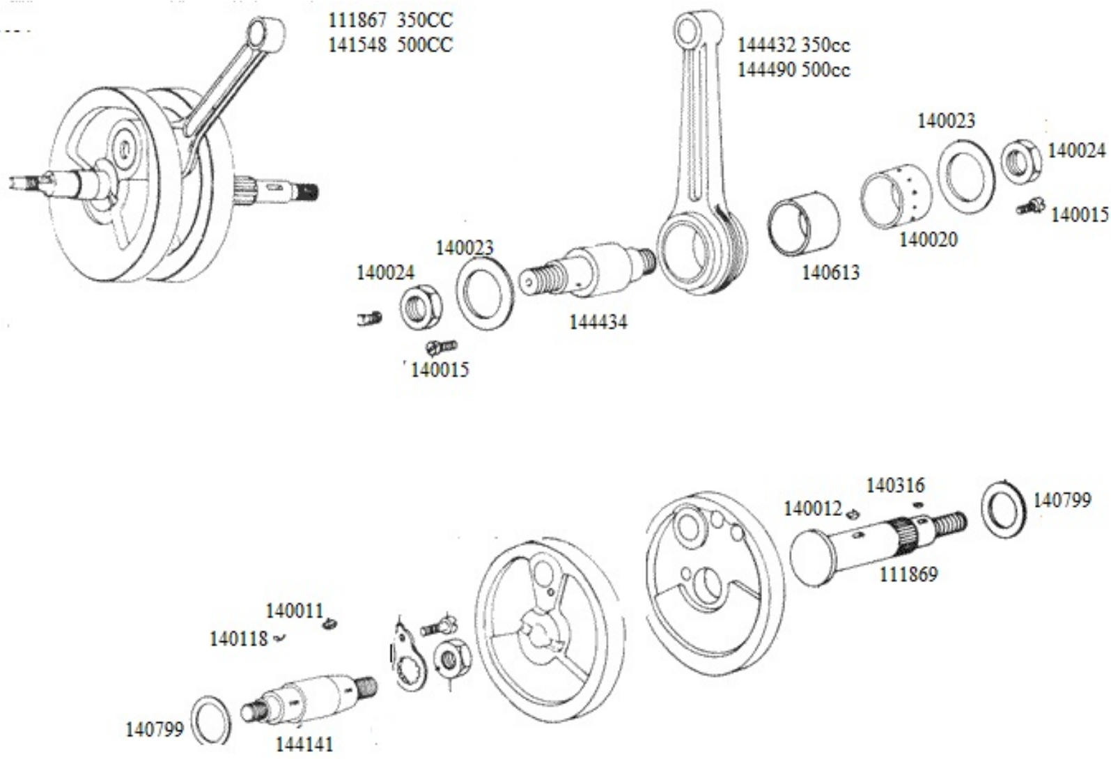
BULLET 350cc & 500CC CRANKSHAFT
